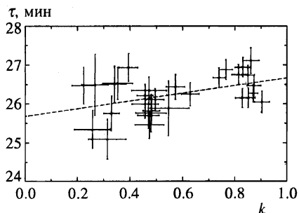
Рис. 4. Экспериментальные точки \tau(k) для экспериментальной серии T и линейная аппроксимация методом максимального правдоподобия
