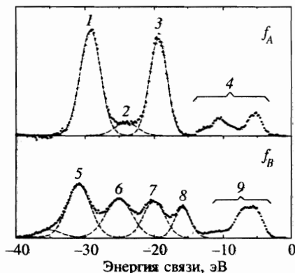
Рис. 6. Чистые спектры f_A и f_B , найденные по серии экспериментальных смешанных спектров R . Обозначения линий: 1 — «6p 1/2 », 2 — «O2s», 3 — «6p 3/2 », 4 — VB, 5 — «6p 1/2 » (1S1u), 6 — «O2s» (2S1u), 7 — «6p 3/2(l) » (1S3u), 8 — «6p 3/2(r) » (3S1u), 9 — VB
