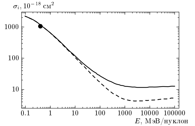
Рис. 1. Зависимость сечения ионизации атома водорода частично ободранными ионами U^{6+} от энергии иона. Сплошная линия — расчетное сечение для протяженного иона, штриховая — сечение ионизации точечным ионом для тех же значений энергии (на нуклон) и заряда, точка — эксперимент [5] (для столкновений C^{6+} + H )
