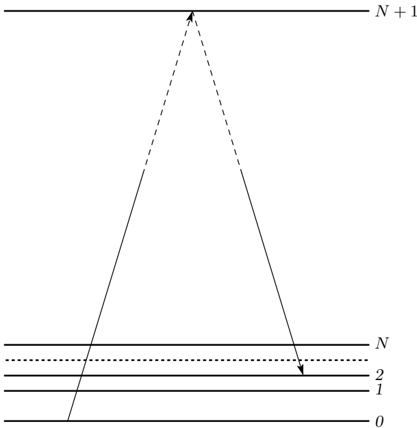
Квантовые уровни молекулы с N нормальными колебательными модами; 0 — основной электронный уровень молекулы; 1, 2, . . . , N — колебательные подуровни; N+1 соответствует возбужденным электронным состояниям. Стрелками изображен один из возможных двухфотонных переходов, штриховые линии указывают на отсутствие в спектре возбуждающих предельно коротких импульсов фурье-компонент, резонансных электронно-оптическим переходам
