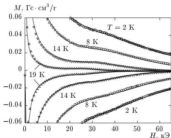
Рис. 3. Участок петель намагниченности V_{0.6}K_{0.4}BiO_3 в районе вторичного пика при различных T . Точки — эксперимент, линии — расчет по ECSM с учетом фазового расслоения (4)
