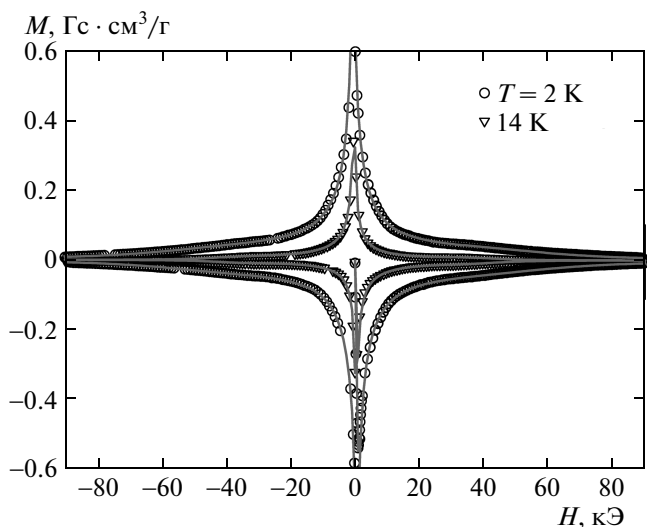
Рис. 2. Петли намагниченности V_{0.6}K_{0.4}BiO_3 при T = 2.14 К. Точки — эксперимент, линии — расчет по ECSM с учетом фазового расслоения (4)
