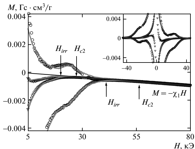
Рис. 4. Участки петель намагниченности V_{0.6}K_{0.4}BiO_3 при T = 21 К (○), T = 25 К (▽). Прямая линия — диамагнитный вклад V_{0.6}K_{0.4}BiO_3 . Показаны примеры определения H_{c2} и H_{irr} . Сплошные линии — расчет по ECSM с учетом фазового расслоения (4). На вставке: те же зависимости после вычета диамагнитного вклада
