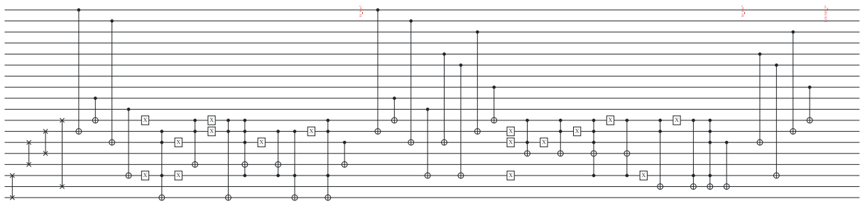
Рис. 6. Третья часть схемы: обратное преобразование второго раунда SDES
