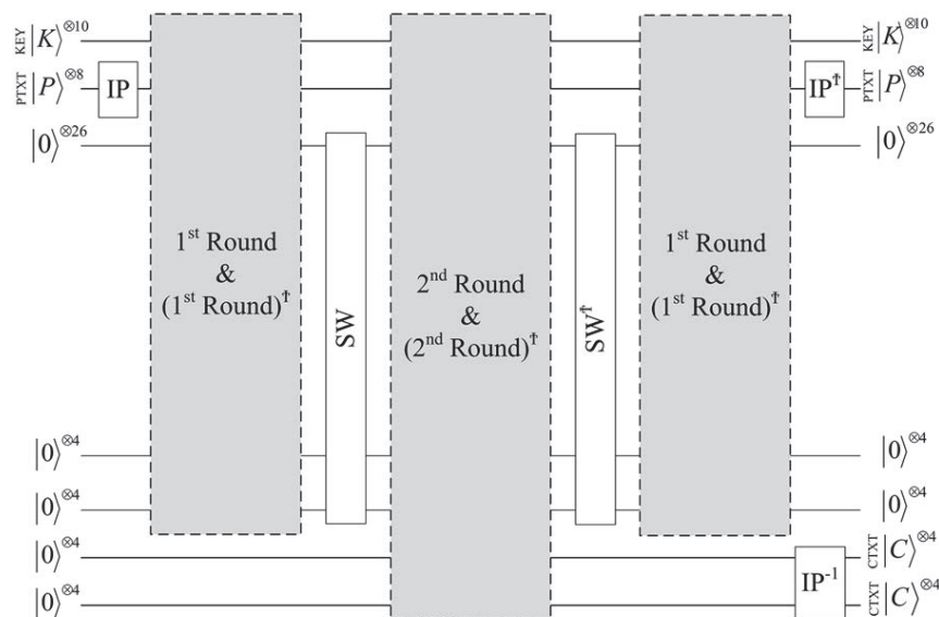
Рис. 2. Реализация SDES в виде квантовой схемы
