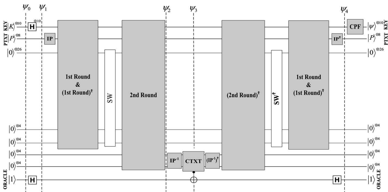
Рис. 3. Квантовая схема одной итерации Гровера
