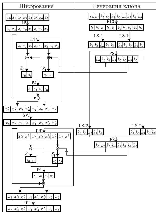
Рис. 1. Схема алгоритма SDES
