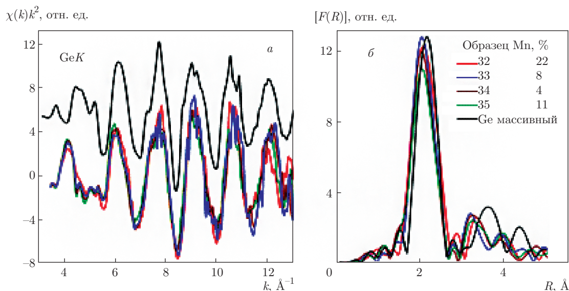
Рис. 3. (В цвете онлайн) a ) Экспериментальные GeK-спектры EXAFS образцов 32–35 с различным содержанием Mn, определенным методом резерфордского обратного рассеяния, и с низкотемпературным (200 °С) защитным слоем Si толщиной 2 нм. б ) Модули фурье-преобразования (радиальные структурные функции без учета фазового сдвига) экспериментальных GeK-спектров EXAFS образцов 32–35
