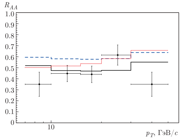
Рис. 3. Импульсная зависимость фактора ядерной модификации заряженных B -мезонов в соударениях РbРb при энергии \sqrt{s_{NN}} = 5.02 ТэВ для области быстрот |y| < 2.4 . Точки — данные CMS [27], гистограммы — результаты моделирования HYDJET++ (сплошная гистограмма — ядерное экранирование и потери энергии включены; штриховая гистограмма — ядерное экранирование и радиационные потери включены, столкновительные потери выключены; пунктирная гистограмма — ядерное экранирование и столкновительные потери включены, радиационные потери выключены)
