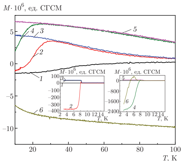
Рис. 24. Зависимость магнитного момента структуры Nb/Ni 0.81 Cu 0.19 (2) от температуры в режимах ZFC и FC спустя 3.5 мес. после изготовления: 1 — ZFC, H = 0; 2 — ZFC, H = 25 Э; 3 — FC, H = 25 Э; 4 — ZFC, H = 150 Э; 5 — FC, H = 150 Э; 6 — ZFC, H = 5 кЭ. На левой вставке: 1 — ZFC, H = 0; 2 — ZFC, H = 25 Э; 3 — FC, H = 25 Э. На правой вставке: 1 — ZFC, H = 150 Э; 2 — FC, H = 150 Э; 3 — ZFC, H = 5 кЭ
