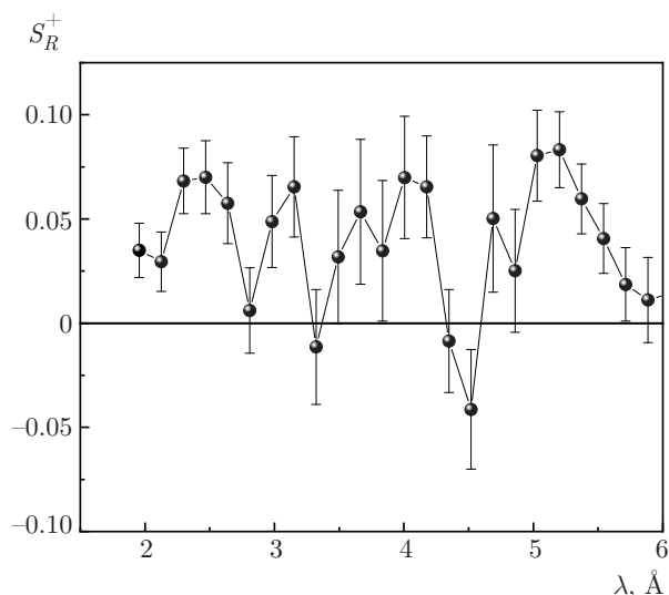
Рис. 29. Асимметрия отражения нейтронов в «плюс»-спиновом состоянии S_R^+ (5 K, 10 K) для структуры Ni_{0.65}Cu_{0.35}(4)
