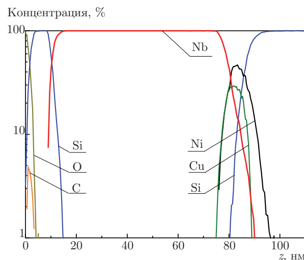
Рис. 13. Пространственные профили элементов структуры Nb/Ni 0.65 Cu 0.35 (4) при t_L = 15 мес.
