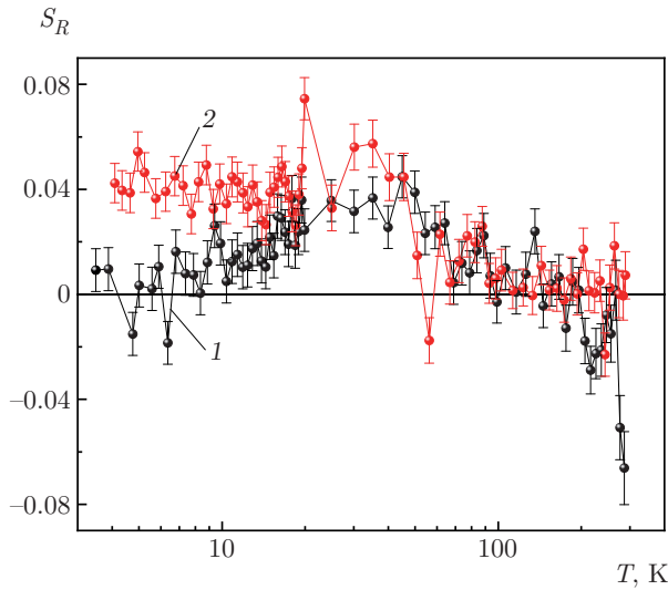
Рис. 27. Зависимости поляризационной асимметрии зеркального отражения нейтронов в режимах ZFC (1) и FC (2) в магнитном поле H = 70 Э для структуры Nb/Ni_{0.81}Cu_{0.19} (2). Для температуры блокировки получено значение 25 К, которое в отличие от данных рассеяния нейтронов меньше магнитометрического значения 29 К
