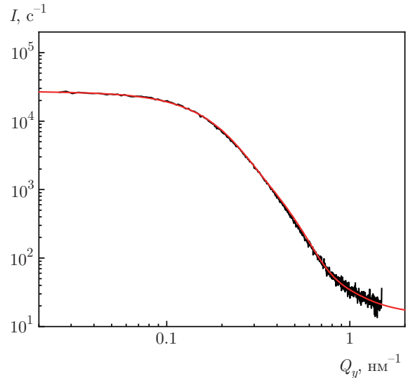
Рис. 2. (В цвете онлайн) Экспериментальная (черный цвет) и расчетная (красный цвет) зависимости интенсивности рассеяния синхротронного излучения для \theta = 10 мрад
