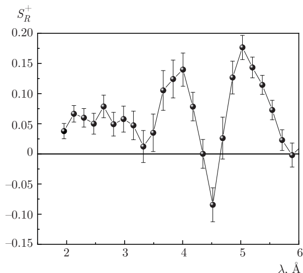
Рис. 30. Асимметрия отражения нейтронов в «плюс»-спиновом состоянии S_R^+ (1.5 K, 10 K) для структуры Ni_{0.65}Cu_{0.35}(4)
