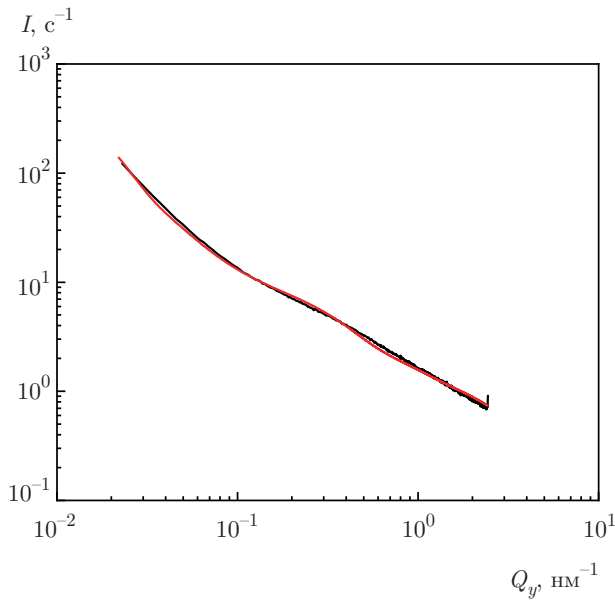
Рис. 17. (В цвете онлайн) Экспериментальная (черный цвет) и расчетная (красный цвет) зависимости интенсивности рассеяния синхротронного излучения для структуры Nb/Ni 0.81 Cu 0.19 (2) при \theta = 5 мрад. Значения параметров, полученные в результате подгонки экспериментальных данных: G_1 = 500, R_1 = 100, B_1 = 0.06, P_1 = 2, G_2 = 5, R_2 = 5.1, B_2 = 0, P_2 = 0, G_3 = 3, R_3 = 2, B_3 = 2.1, P_3 = 1.2, C = 0.028
