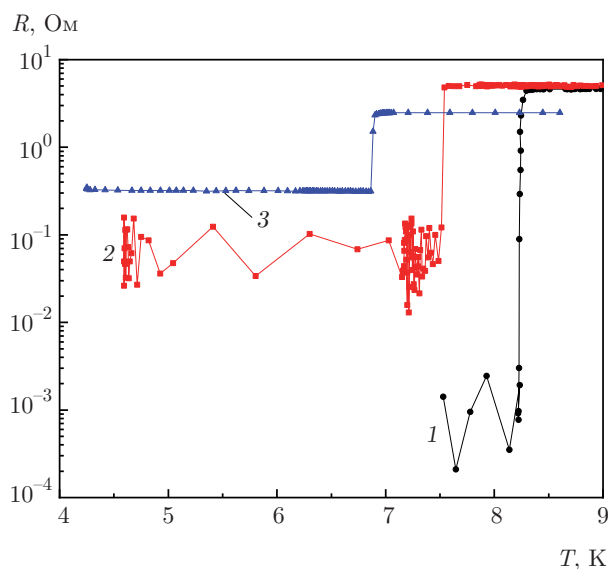
Рис. 14. Зависимость сопротивления структуры Nb/Ni 0.81 Cu 0.19 (4) от температуры при H = 0 : спустя две недели после изготовления структуры (1), спустя один месяц (2) и спустя два месяца (3)
