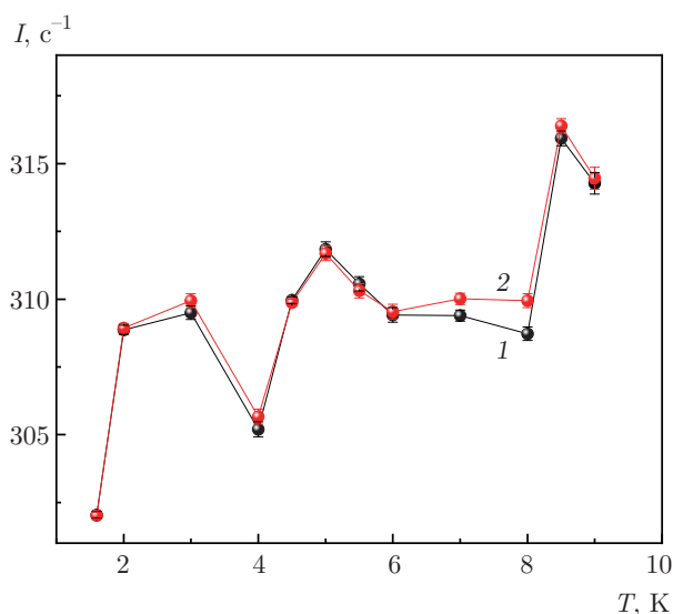
Рис. 31. Температурная зависимость интенсивности нейтронов для структуры Nb/Ni 0.81 Cu 0.19 (4) в магнитное поле 25 Э при длине волны нейтронов \lambda = 2 Å и поляризации P_0 = +1 (1) и P_0 = -1 (2)
