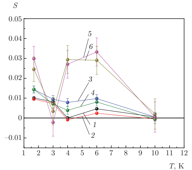
Рис. 10. Зависимость коэффициента рассеяния нейтронов S(T) для структуры V/FeV/V/FeV/Nb при t_L = 3.5 г. для H = 28 \text{ Э} : \lambda = 2 \pm 0.2 \text{ \AA} , P_0 = +1 (1); \lambda = 2 \pm 0.2 \text{ \AA} , P_0 = -1 (2); \lambda = 4.6 \pm 0.46 \text{ \AA} , P_0 = +1 (3); \lambda = 4.6 \pm 0.46 \text{ \AA} , P_0 = -1 (4); \lambda = 7.2 \pm 0.72 \text{ \AA} , P_0 = +1 (5); \lambda = 7.2 \pm 0.72 \text{ \AA} , P_0 = -1 (6)
