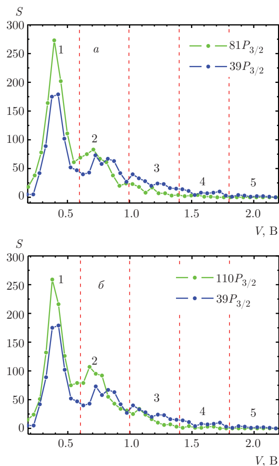
Рис. 7. (В цвете онлайн) Сравнение гистограмм выходных импульсов умножителя ВЭУ-6 для разного числа N регистрируемых ридберговских атомов при настройке на центры линий лазерных переходов в не взаимодействующее состояние 39P_{3/2} и во взаимодействующее состояния 81P_{3/2} (а) и 110P_{3/2} (б). Наличие частичной дипольной блокады для высоких ридберговских состояний 81P_{3/2} и 110P_{3/2} уменьшает амплитуды сигналов для N = 3-5 и увеличивает их для N = 1, 2
