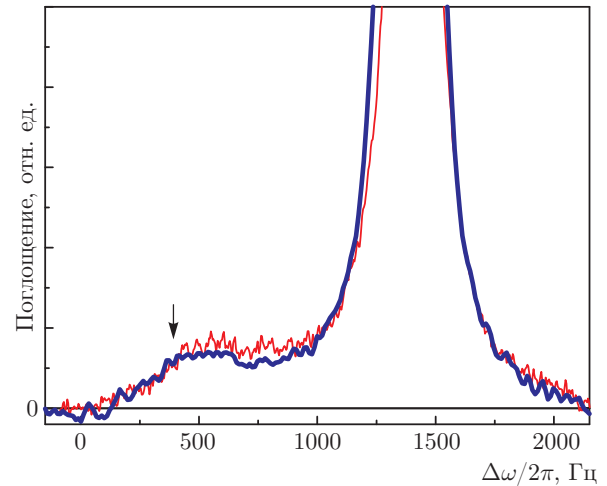
Рис. 9. (В цвете онлайн) Спутная и основная линии непрерывного ЯМР в образце нафен-910 при наличии полуквантовых вихрей (толстая линия) и при наличии спиновых вихрей (тонкая линия). P = 23.6 бар, \mu = 40^\circ , \omega/2\pi = 546 кГц, T \approx 0.4T_c , T_{ca} \approx 0.68T_c . Стрелка указывает на ожидаемое положение спутных пиков при \lambda = 1
