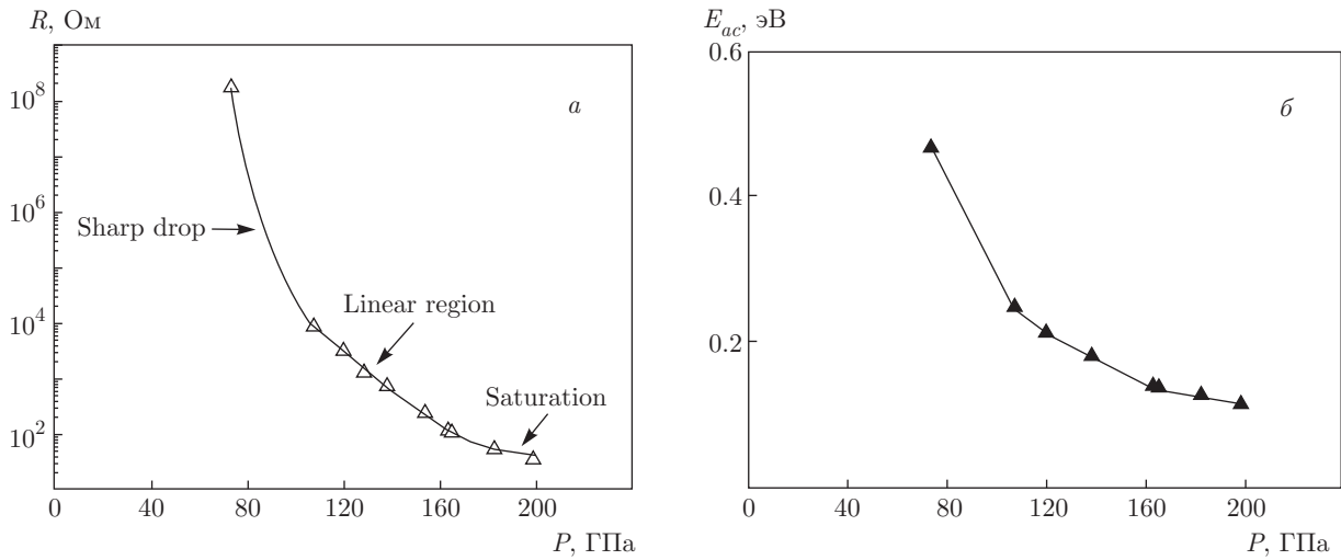
Рис. 10. Зависимости электросопротивления монокристалла FeBO 3 (а) и энергии активации (б) от давления при T = 300 К (из работы [66])
