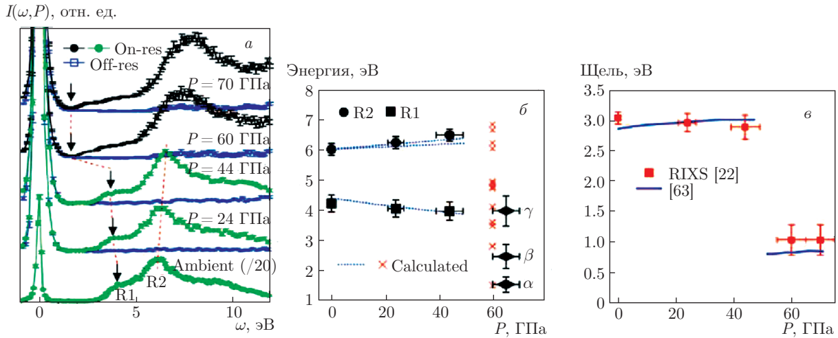
Рис. 8. (В цвете онлайн) Изменения спектров RIXS с ростом давления, непосредственно показывающие изменения диэлектрической щели (стрелки) (а), рассчитанные из этих спектров энергии возбуждений Мотта – Хаббарда (б) и величина диэлектрической щели по данным RIXS и оптических спектров поглощения [63] (в) (из работы [22])
