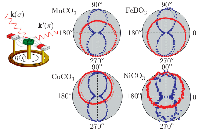
Рис. 2. (В цвете онлайн) Схема рентгеновского дифракционного эксперимента (схематический вид и основные результаты), нормализованные экспериментальные значения интенсивности дифракции в зависимости от величины \eta — угла поворота магнита относительно c -оси кристалла, тонкие сплошные линии — подгонка (из работы [27])
