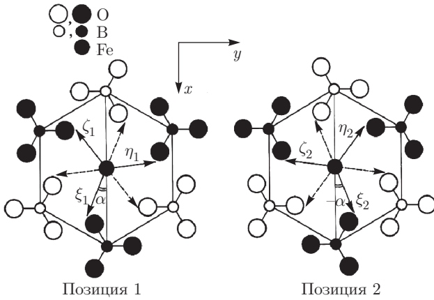
Рис. 3. Схематическое распределение «осей кубического кристаллического поля» для двух неэквивалентных позиций ионов M^{3+} в решетке MBO_3 . («Темные ионы» BO_3^{3-} расположены выше плоскости рисунка, светлые — ниже). (Из работы [15])
