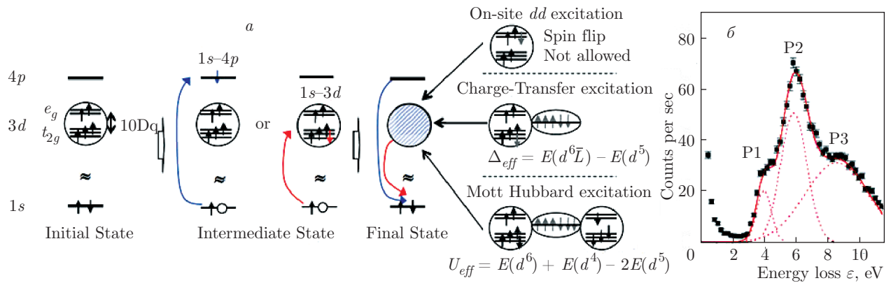
Рис. 4. а) Схема формирования К-края Fe резонансного неупругого рентгеновского рассеяния. б) Спектр предкраевых особенностей в FeVO 3 . (Из работы [21])
