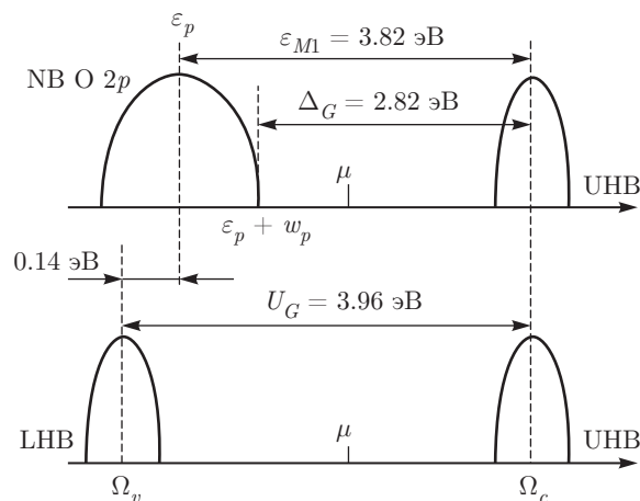
Рис. 6. Схема электронной структуры FeBO 3 , полученная на основе экспериментов RIXS, сверху показаны вклады возбуждений с переносом заряда, внизу — вклады от возбуждений Мотта-Хаббарда (из работы [21])
