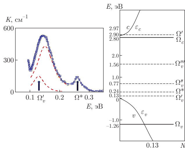
Рис. 7. ИК-спектры FeBO 3 при комнатной температуре (а) и плотность одночастичных электронных состояний с указанием виртуальных уровней (б). (Из работы [20])
