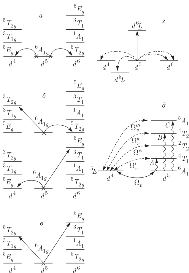
Рис. 5. Схема многоэлектронных возбуждений для FeBO 3 . а-в) Мотт-хаббардовские возбуждения d_i^5 d_j^5 \rightarrow d_i^4 d_j^6 , ассоциированные с предкраевыми особенностями P1, P2, P3 в спектрах RIXS. г) Два типа возбуждений с переносом заряда (сплошные и штриховые линии) и возбуждения Мотта-Хаббарда (штрихпунктирные линии) (из работы [21]). д) Виртуальные одноэлектронные состояния, обусловленные возбуждениями из незаполненного термина d^4 в незаполненные возбужденные термы d^5 (из работы [20])
