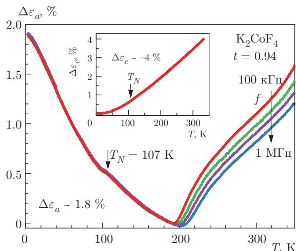
Рис. 6. (В цвете онлайн) Температурная зависимость относительной диэлектрической проницаемости \epsilon_a вдоль оси a в слоистом тетрагональном фтороперовските \text{K}_2\text{CoF}_4 . На вставке показана зависимость \epsilon_c(T) вдоль оси c , и в этом случае в противоположность \epsilon_a никакой частотной дисперсии не было обнаружено
