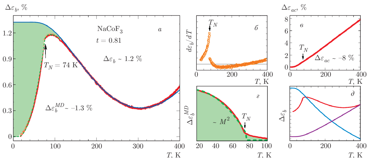
Рис. 2. (В цвете онлайн) Температурные зависимости относительной диэлектрической проницаемости ромбического фторперовскита \text{NaCoF}_3 \epsilon_b вдоль оси b (а); производной d\epsilon_b/dT , на которой четко проявляется максимум, соответствующий T_N (б); диэлектрическая проницаемость \epsilon_{ac} в направлении [101] (в); спонтанный МД-эффект \Delta\epsilon_b^{MD} вдоль оси b (г); разложение \epsilon_b (красная линия) на составляющие, описываемые функциями Барретта (б) — синяя линия и Эйнштейна (5) — фиолетовая линия (д)
