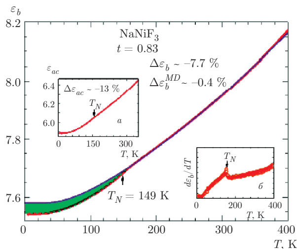
Рис. 3. (В цвете онлайн) Температурная зависимость диэлектрической проницаемости \varepsilon_b вдоль оси b в ромбическом фтороперовските \text{NaNiF}_3 . На вставках показаны зависимость \varepsilon_{ac}(T) , измеренная в направлении [101] (а) и производная d\varepsilon_b/dT , на которой четко виден максимум, соответствующий T_N (б)
