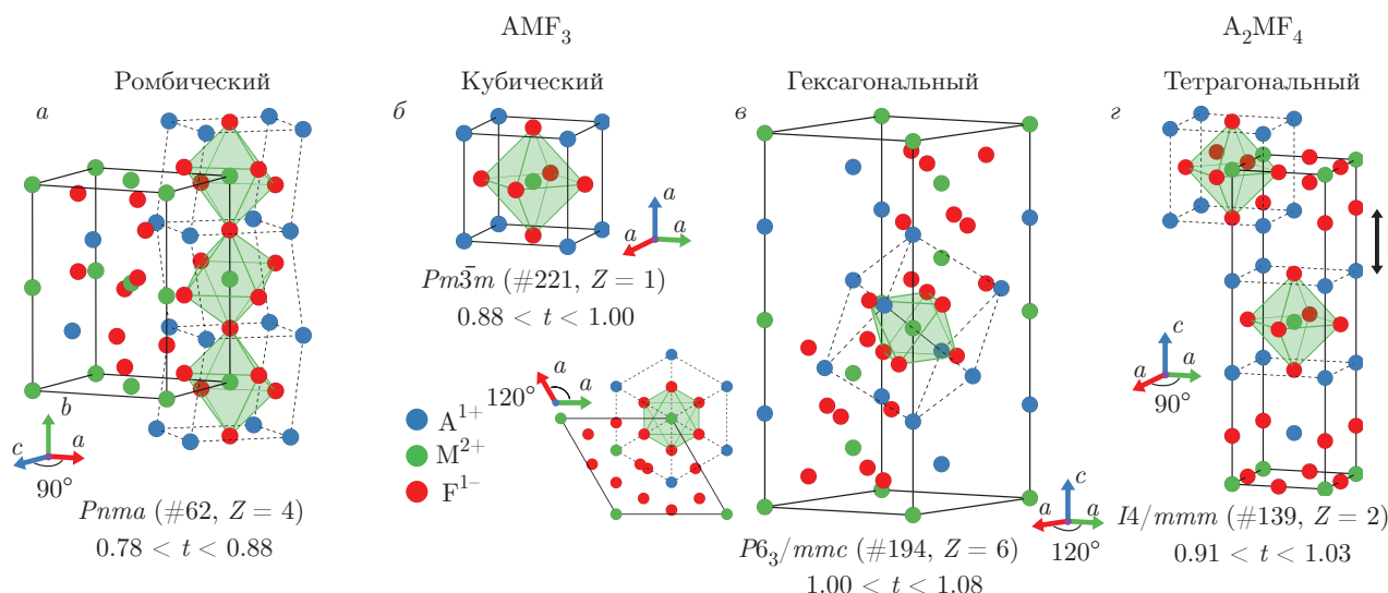
Рис. 1. (В цвете онлайн) Кристаллические структуры ромбического (а), кубического (б), гексагонального (в) фторперовскитов AMF_3 и тетрагонального слоистого фторперовскита A_2MF_4 (д, черной стрелкой показано направление чередования перовскитных слоев). Диапазоны значений коэффициента толерантности t для соответствующих структур показаны под рисунками. Изображения кристаллических структур получено с использованием программы VESTA [53]
