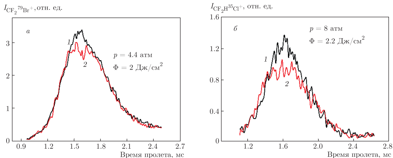
Рис. 2. (В цвете онлайн) Временные зависимости величин ионных сигналов CF_2^{79}Br^+ (а) и CF_2H^{35}Cl^+ (б) без облучения молекулярного потока в скачке уплотнения (1) и в случае облучения CO_2 -лазером (2) на линии 9R(30) (на частота 1084.635 см -1 ) при плотностях энергии 2 Дж/см 2 (а) и 2.2 Дж/см 2 (б). Давление CF_3Br над соплом 4.4 атм (а). Давление смеси CF_2HCl/CF_3Br = 1/1 над соплом 8 атм (б). Длительности импульсов открывания сопла 350 мкс (а) и 475 мкс (б)
