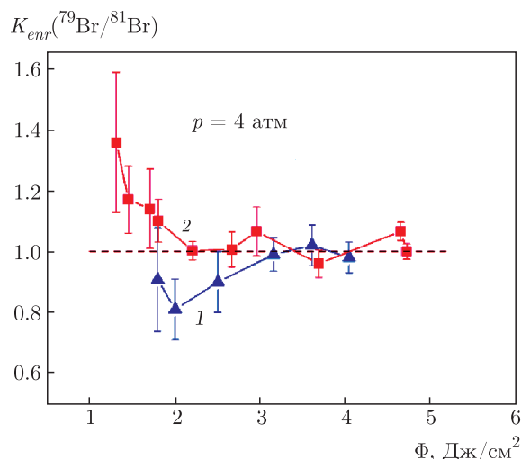
Рис. 5. Зависимости коэффициентов обогащения K_{enr}(^{79}\text{Br}/^{81}\text{Br}) в продукте \text{Br}_2 от плотности энергии возбуждающего излучения в случае облучения молекул \text{CF}_3\text{Br} в потоке, падающем на поверхность (1), и в скачке уплотнения (в ударной волне) (2). Молекулы возбуждались на линии 9R(30) лазера (на частоте 1084.635\text{ см}^{-1} ). Давление газа над соплом 4 атм. Длительность импульса открывания сопла 350 мкс
