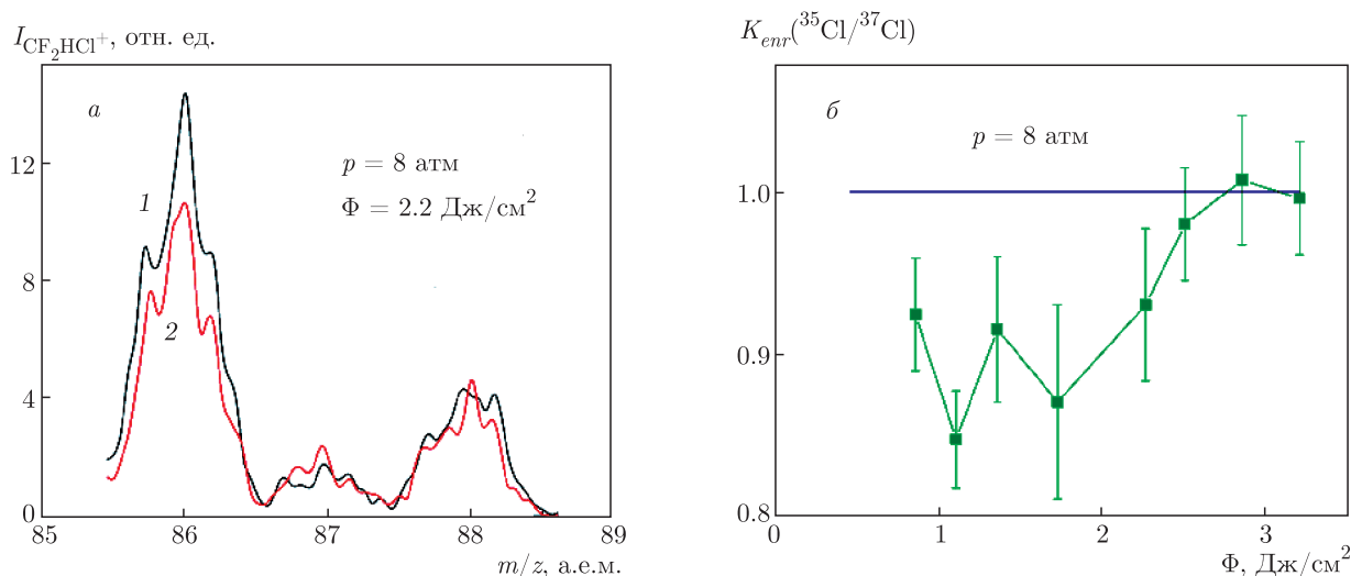
Рис. 7. а) Масс-спектры молекул CF_2HCl ( m/z = 86, 87, 88 ) до облучения (1) и после облучения смеси CF_2HCl/CF_3Br = 1/1 в ударной волне (2). Молекулы возбуждались на линии 9R(30) лазера (на частоте 1084.635\text{ см}^{-1} ) при плотности энергии 2.2\text{ Дж/см}^2 . б) Зависимость коэффициента обогащения K_{enr}(^{35}Cl/^{37}Cl) в остаточном газе CF_2HCl при облучении смеси молекул CF_2HCl/CF_3Br = 1/1 на линии 9R(30) лазера. В обоих случаях (а и б) давление газа над соплом 8 атм, длительность импульса открывания сопла 475 мкс
