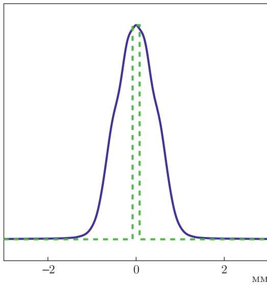
Рис. 3. Профиль изображения щели на рис. 2, ср. с рис. 5 из [38], (сплошная линия) и профиль распределения прозрачностей самой щели (штриховая)
