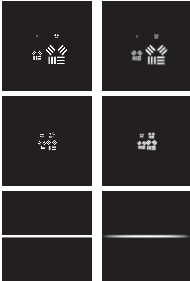
Рис. 4. Моделирование формирования квантовых фантомных изображений оптических мир и щели согласно формуле (12). Расстояния между щелями мир 0.01, 0.02, 0.05, 0.1 мм (верхняя пара изображений; 50, 25, 10 и 5 штрихов на миллиметр), 0.02, 0.03, 0.04, 0.05 мм (средняя пара изображений; 25, 16.7, 12.5 и 10 штрихов на миллиметр). Ширина щели 0.16 мм. В левом столбце распределения прозрачностей объектов T(\cdot) , в правом — корреляционные функции G(\cdot)
