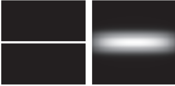
Рис. 2. Моделирование формирования квантовых фантомных изображений согласно формуле (12). Размер изображений 6 × 6 мм. Слева — распределение прозрачности объекта T(\cdot) (щель шириной 0.16 мм), справа — корреляционная функция G(\cdot)
