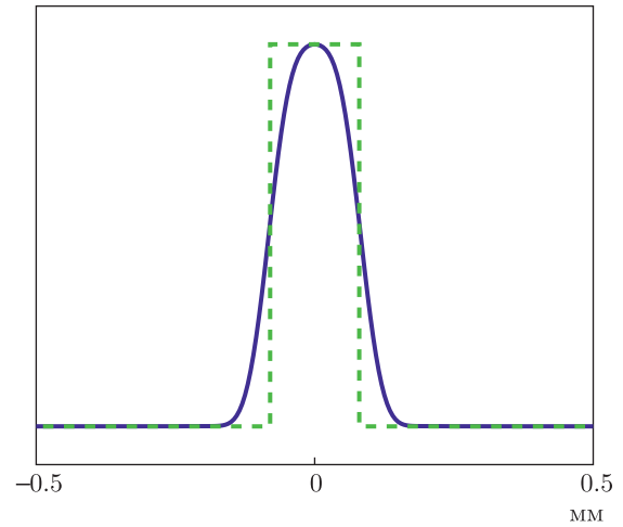
Рис. 5. Профиль изображения щели на рис. 4 (сплошная линия) и профиль распределения прозрачностей самой щели (штриховая)
