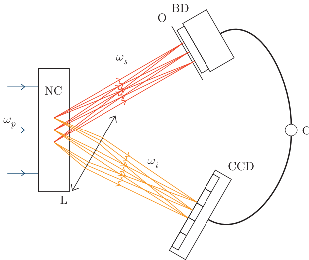
Рис. 1. Формирование квантового фантомного изображения. NC — нелинейный кристалл, \omega_p — луч накачки, \omega_s и \omega_i — лучи запутанных фотонов (которые расходятся вследствие использования неколлинеарного параметрического рассеяния), O — исследуемый объект, BD — собирающий детектор в объектном канале, L — линза, CCD — матрица датчиков в восстанавливающем канале, C — коррелятор интенсивностей (схема совпадений)
