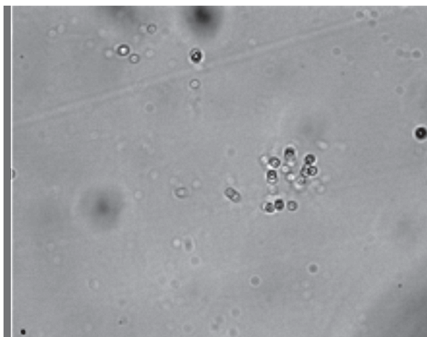
Рис. 3. Микрофотография кольцевой структуры протонных треков на поверхности детектора. Al-фильтр перед детектором имеет толщину 77 мкм. Размер кадра равен 120 \times 90 \text{ мкм}^2
