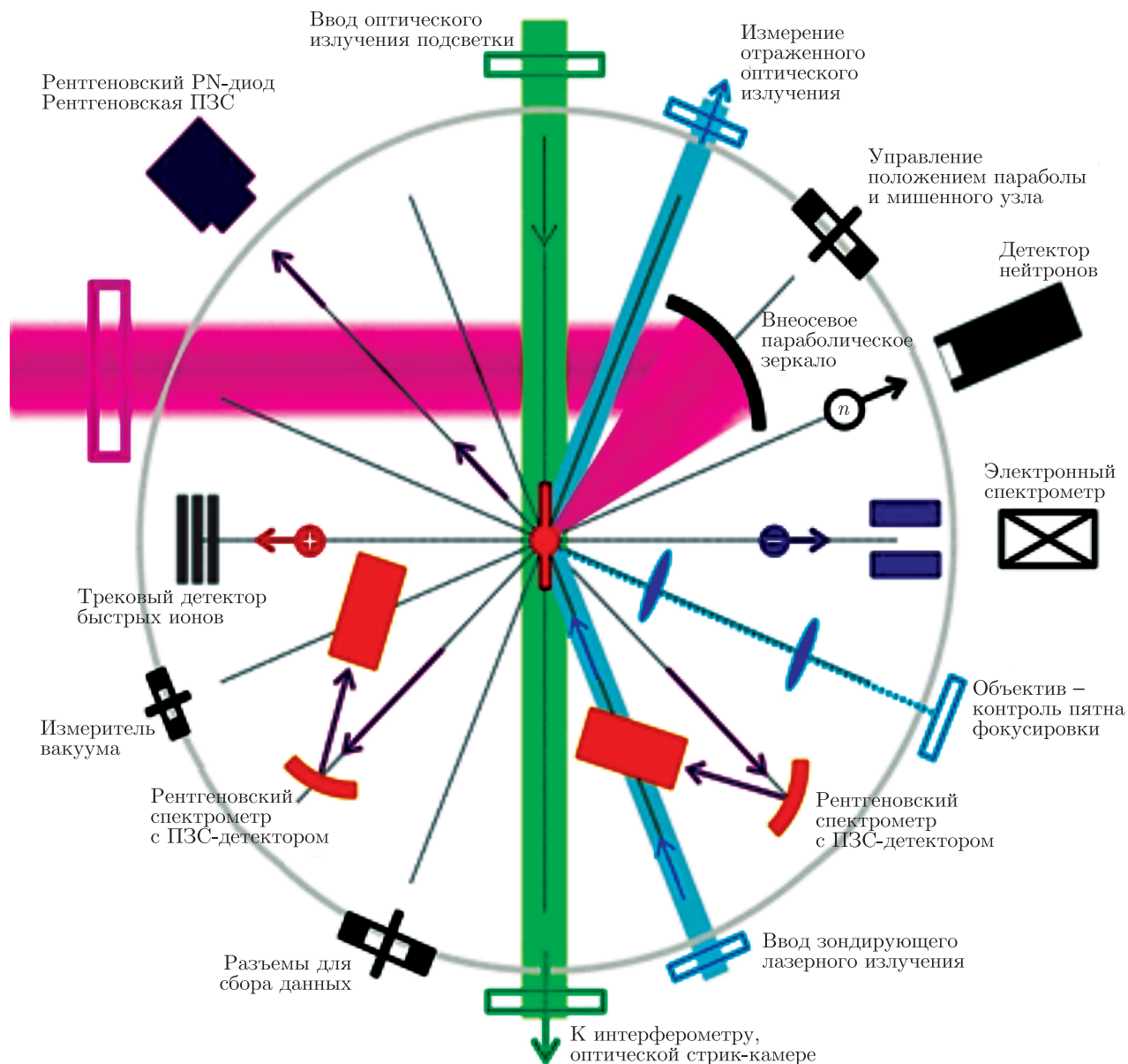
Рис. 1. Схема измерительной аппаратуры и лазерного пучка
