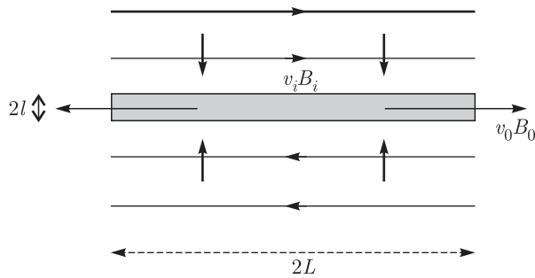
Рис. 6. Модель Свита–Паркера
