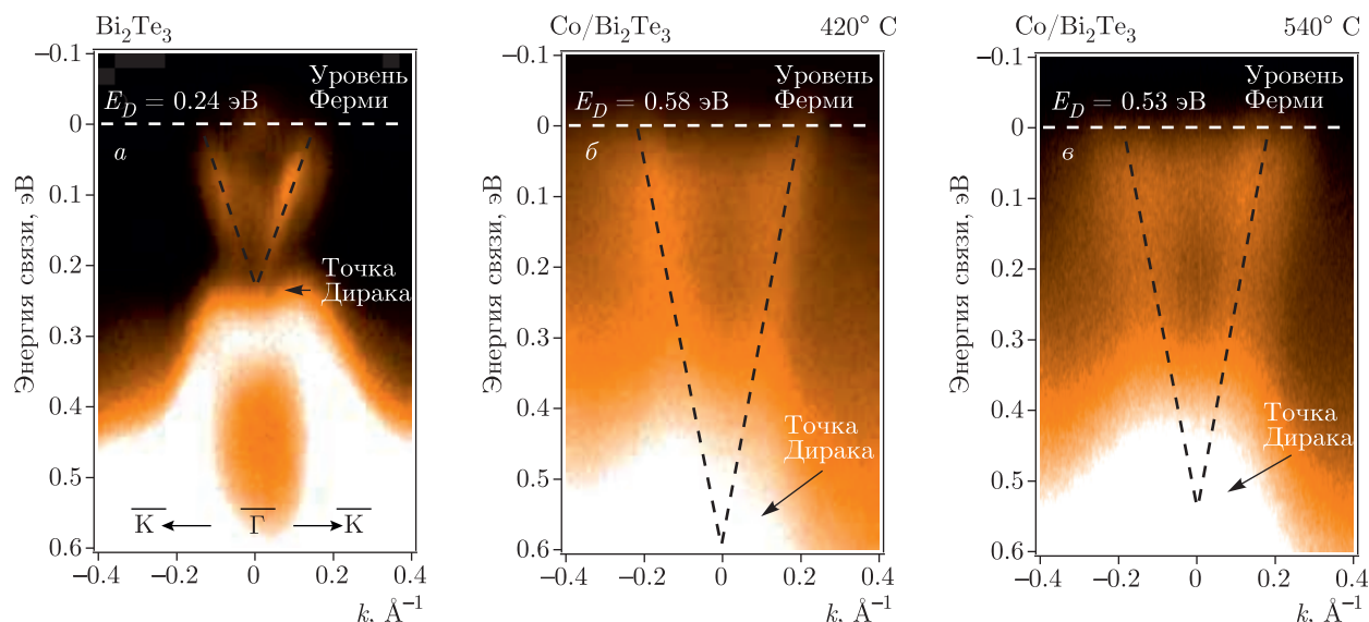
Рис. 1. Спектры ФЭСУР для ТИ \text{Bi}_2\text{Te}_3 : a — чистого, б — после напыления на поверхность слоя Со толщиной 2 \text{ \AA} с одновременным прогревом до T = 420 \text{ }^\circ\text{C} , в — после напыления на поверхность еще одного слоя Со толщиной 1 \text{ \AA} с одновременным прогревом до T = 540 \text{ }^\circ\text{C} , h\nu = 21.2 \text{ эВ}
