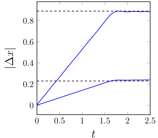
Рис. 4. Сдвиги центров тяжести облаков от их положений в отсутствие взаимодействия, полученные численным решением уравнений для газа Чаплыгина при начальных значениях параметров f_{10} = 0.05 , f_{20} = 0.1 , \kappa_1 = 1.3 , \kappa_2 = 2.5 , l = 10 . В момент T = 1.6 разделения они принимают теоретические значения, даваемые формулами (50).
