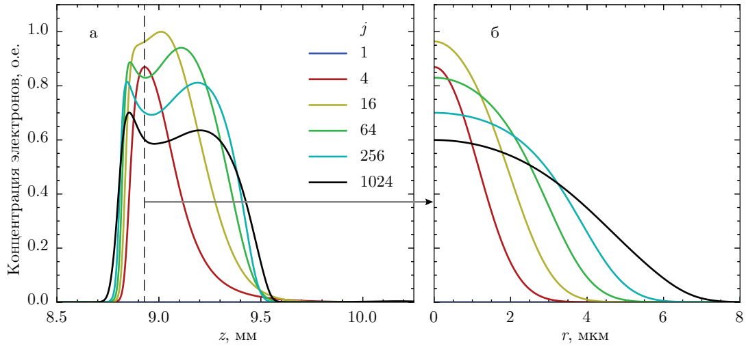
Рис. 5. (В цвете онлайн) Распределения в LiF относительной концентрации электронов \rho_e^j(r = 0, z)/\rho_{e\max} на оси (а) и в поперечном сечении \rho_e^j(r, z^*)/\rho_{e\max} (б) филамента после воздействия j -го импульса. Положение поперечного сечения при z^* = 8.93 мм показано вертикальной штриховой линией на рис. а
