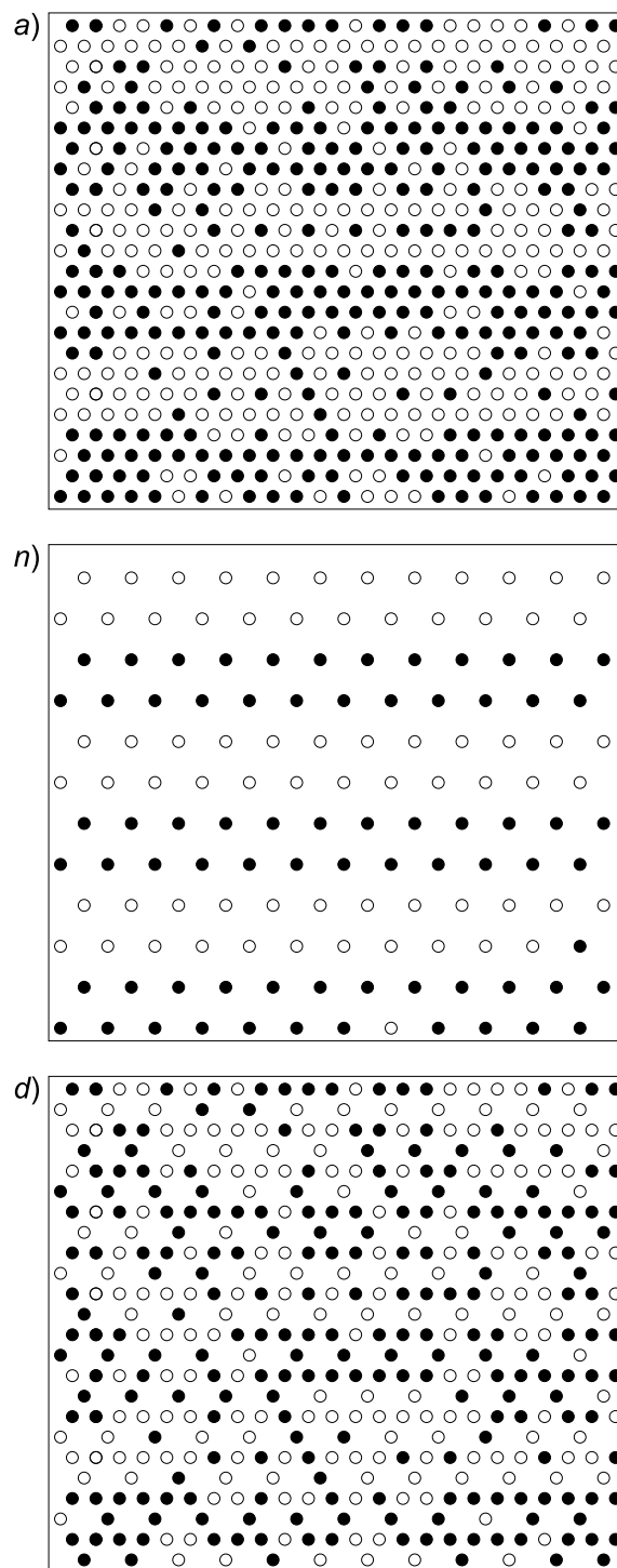
Рис. 9. Равновесная конфигурация всех (a), узловых (n) и декорированных (d) спинов для J_d = 0.5 при температуре T = 1.49
