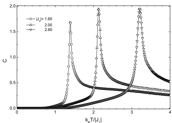
Рис. 11. Зависимость теплоемкости от температуры при различных значениях обменного взаимодействия |J_d| > 1.4
