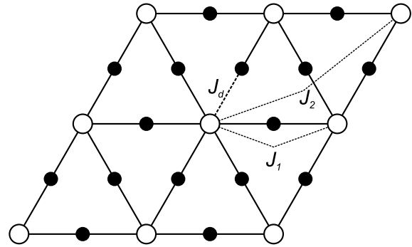
Рис. 1. Декорированная модель Изинга на треугольной решетке (○ — узловые спины, ● — декорированные)
