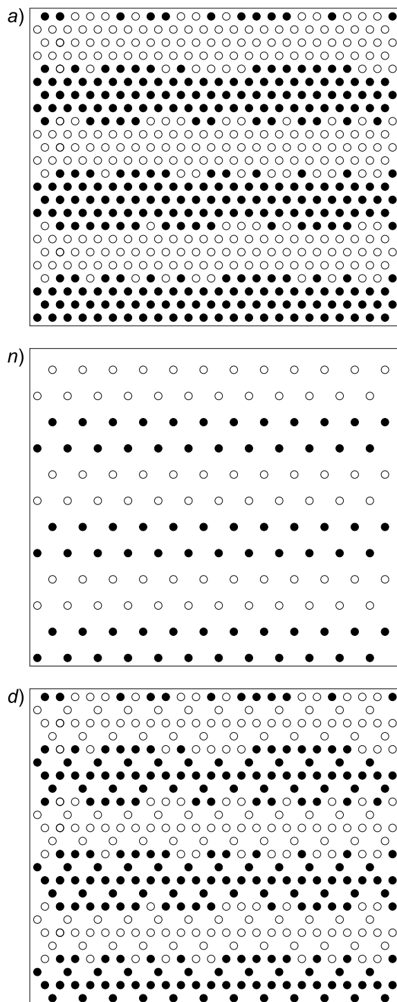
Рис. 4. Конфигурация основного состояния всех (a), узловых (n) и декорированных (d) спинов при J_d = 0.5
