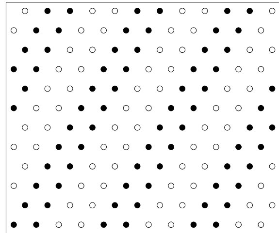
Рис. 2. Страйповое упорядочение в основном состоянии исходной недекорированной решетки. Цветом выделены два противоположных направления спинов
