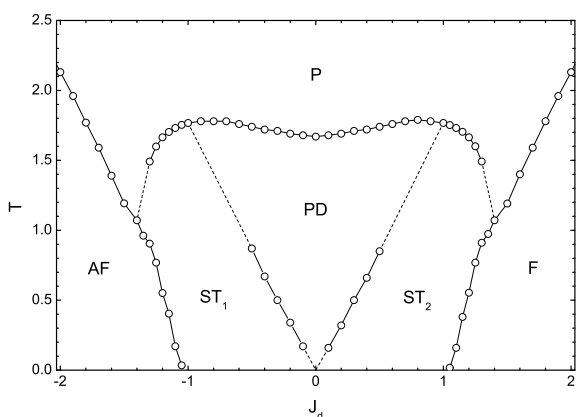
Рис. 12. Фазовая диаграмма, построенная по максимумам теплоемкости для линейного размера L = 24 . AF — антиферромагнитная фаза, F — ферромагнитная, ST — стриповая антиферромагнитная, PD — частично разупорядоченная, P — парамагнитная
