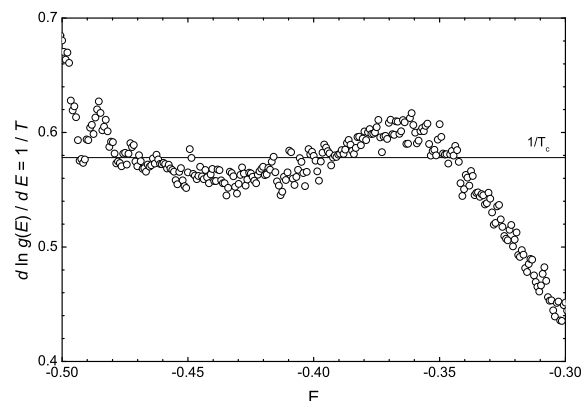
Рис. 14. Зависимость производной логарифма плотности состояний от энергии, L = 12 , J_d = -0.1
