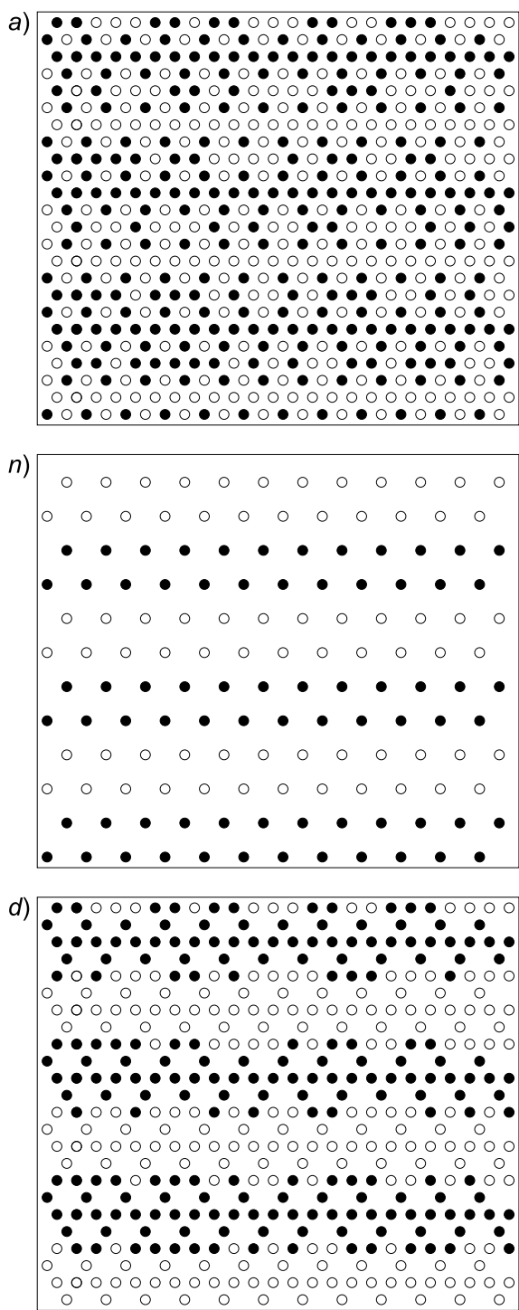
Рис. 3. Конфигурация основного состояния всех (a), узловых (n) и декорированных (d) спинов при J_d = -0.5
