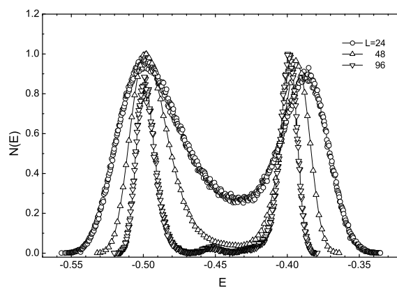
Рис. 15. Гистограмма энергии для различных линейных размеров L , J_d = -0.1
