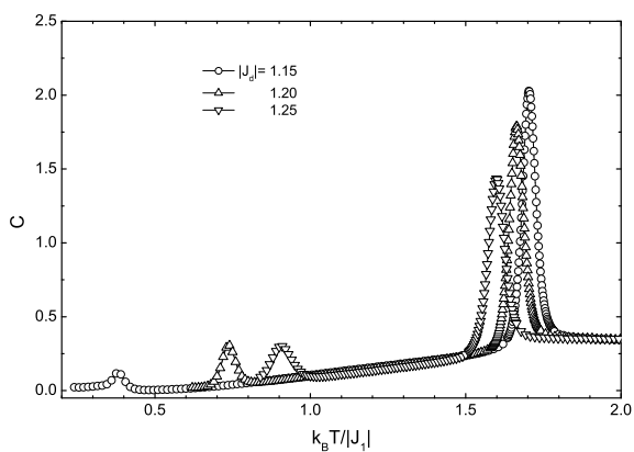
Рис. 10. Зависимость теплоемкости от температуры при различных значениях обменного взаимодействия 1 < |J_d| < 1.3
