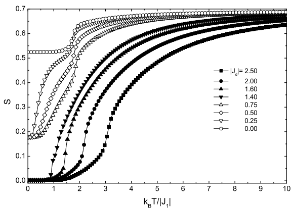
Рис. 7. Зависимость энтропии от температуры при различных значениях обменного взаимодействия J_d
