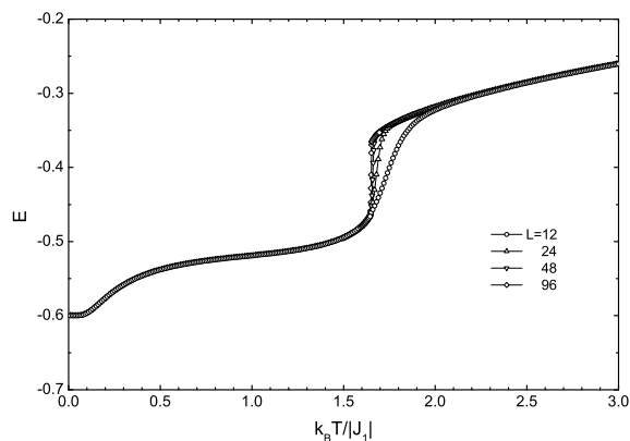
Рис. 13. Зависимость энергии от температуры для различных линейных размеров L при значении обменного взаимодействия |J_d| = 0.1
