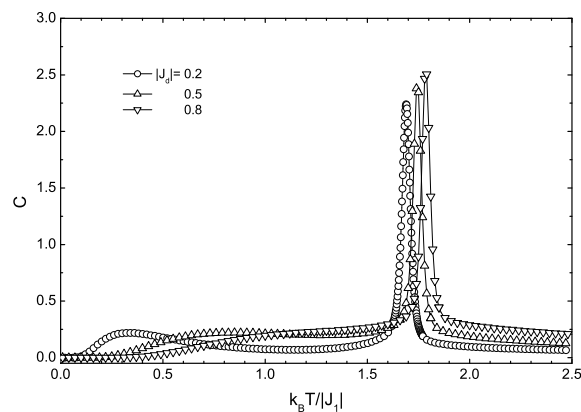
Рис. 8. Зависимость теплоемкости от температуры при различных значениях обменного взаимодействия |J_d| < 1
