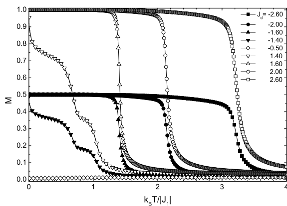
Рис. 5. Зависимость модуля намагниченности от температуры при различных значениях обменного взаимодействия J_d
