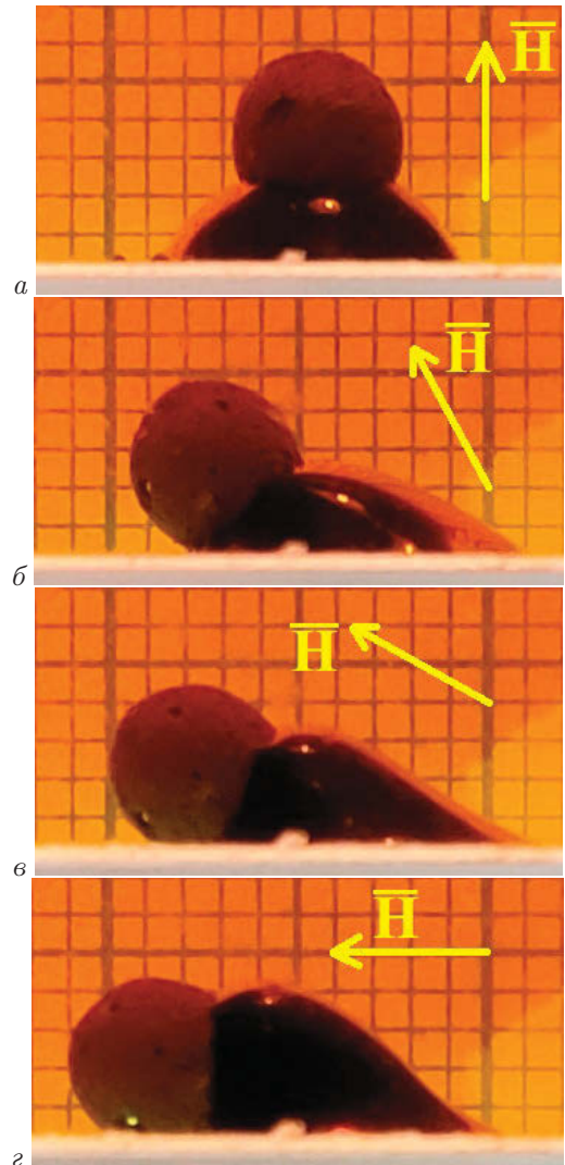
Рис. 9. Фотографии экспериментальных форм поверхности МЖ (вид сбоку) объемом V_f = 0.06 \text{ мл} около намагничивающегося шара при H_\infty = 450 \text{ Э} в эксперименте типа 1 для разных значений параметра \alpha = 0 (а), 30° (б), 60° (в), 90° (г)
