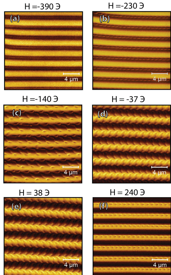
Рис. 3. Эволюция МСМ-изображений доменной структуры при изменении внешнего плоскостного магнитного поля от -390 Э до +240 Э; величина напряженности магнитного поля, при котором выполнено МСМ-измерение, указана возле каждой панели
