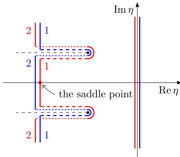
Рис. 2. Контур интегрирования при обратном преобразовании Фурье для нулевого и первого собственных значений, исходные обозначены непрерывными синей и красной линиями. Черными штриховыми линиями обозначены разрывы
