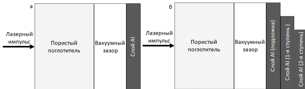
Рис. 2. Схема мишени для измерения одновременности выхода УВ на тыльную поверхность слоя алюминия (а) и схема мишени для исследования временной динамики УВ (б)
