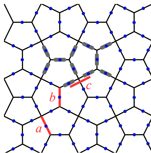
Рис. 1. Схематическое изображение каирской решетки. Синие точки — расположение точечных диполей в исследуемой модели, серые овалы — пример расположения наностроек в соответствующих работах [7, 30, 31]. Наностройки расположены на всех ребрах решетки, на рисунке приведена часть из них. Красные (жирные) линии a , b , c — параметры каирской решетки
