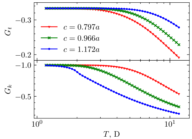
Рис. 7. Температурная зависимость корреляций внутри треугольников G_t и крестов G_k для параметров решетки c = 0.797a, 0.966a, 1.172a и N = 5120 спинов
